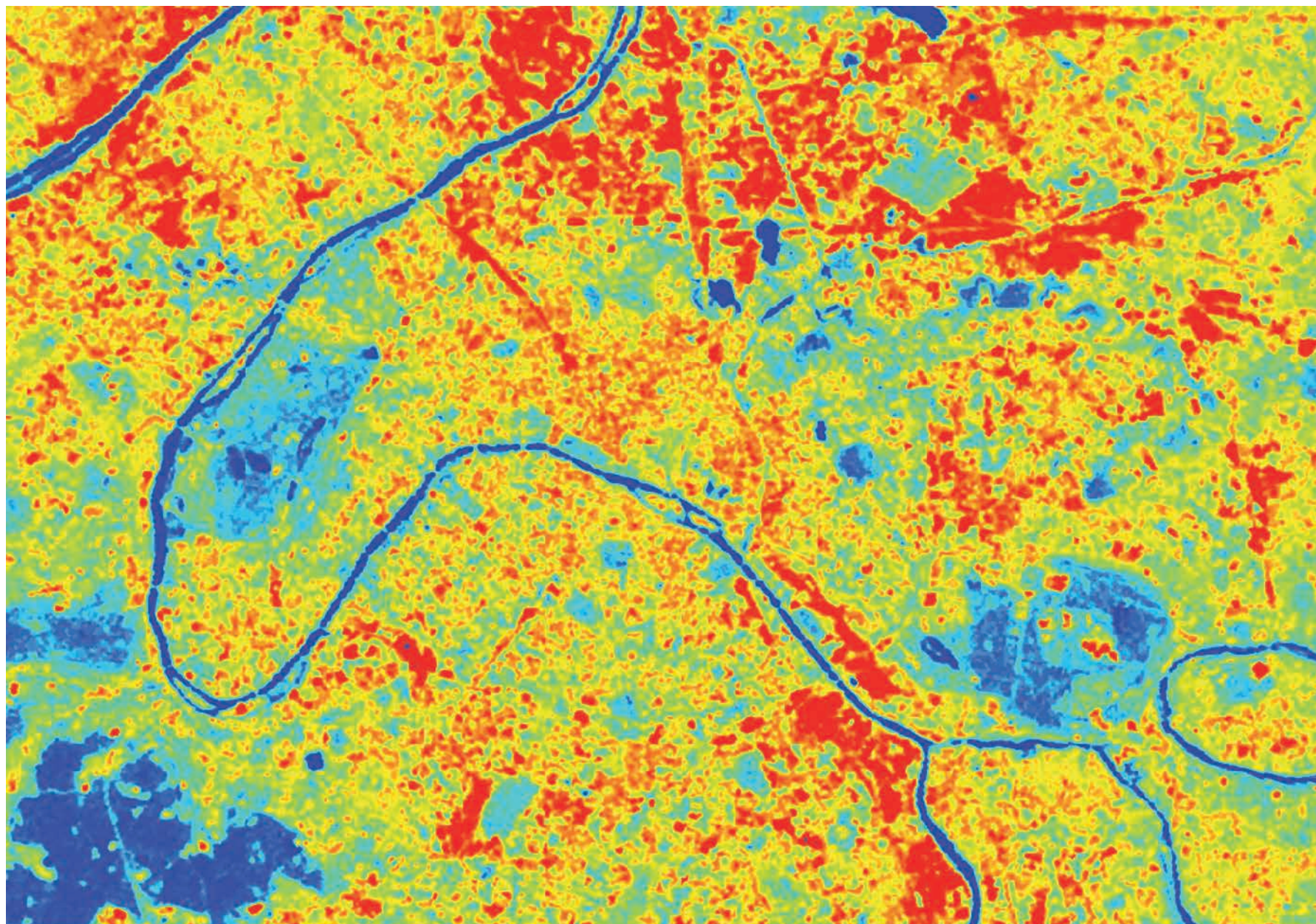
Carte de la thermographie d'été (temps universel, 12h à Paris) du cœur de l'agglomération parisienne montrant le rôle des espaces verts et des cours d'eau pour réduire les îlots de chaleur.
