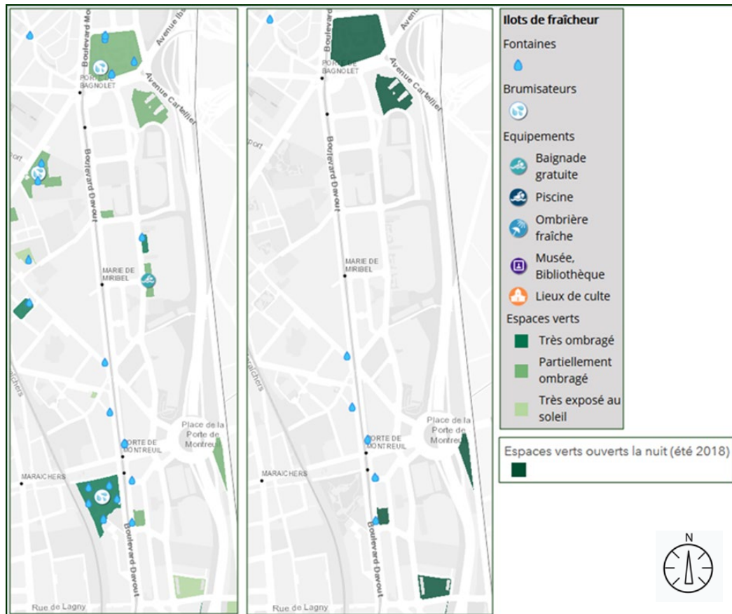
Figure 21 : Cartes des îlots de fraîcheur urbaine (jour et nuit) présents sur le secteur (source : Ville de Paris, 2018)
