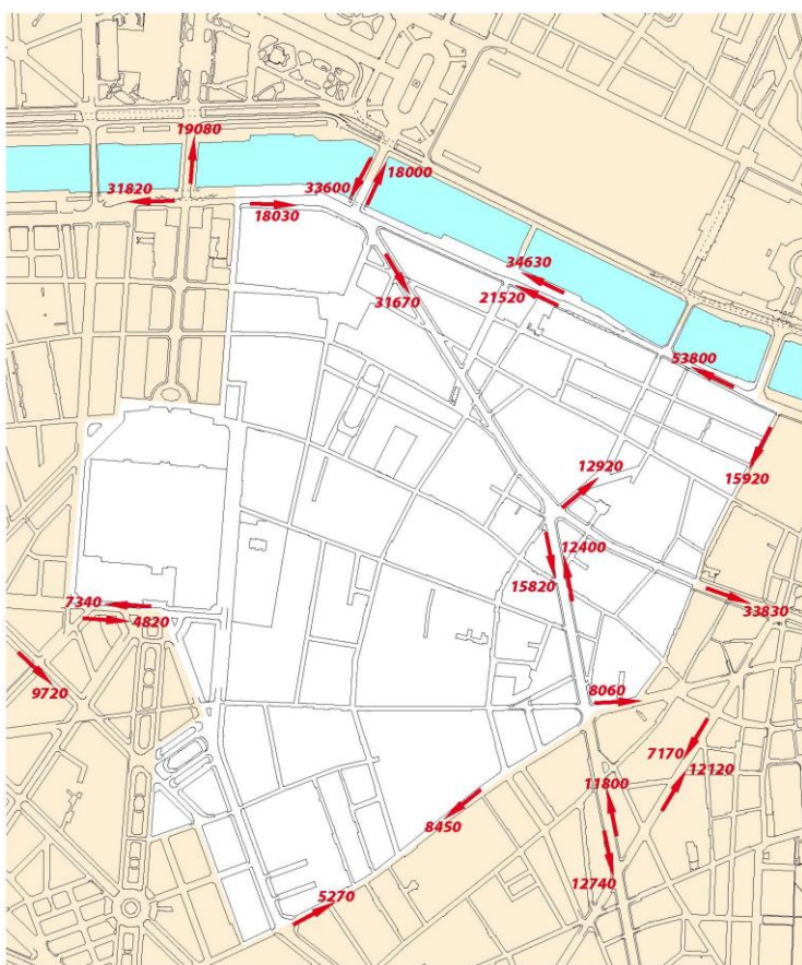
Débits journaliers
