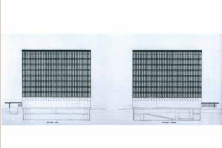
Élévations est et ouest, vers 1957 (© IFA).
