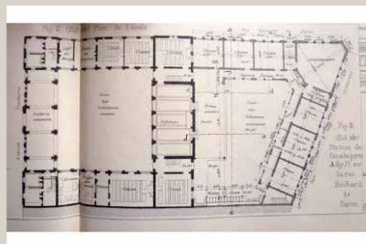
Plan de l'école en 1895 (publié dans Nouvelles annales de la construction , 1895).
