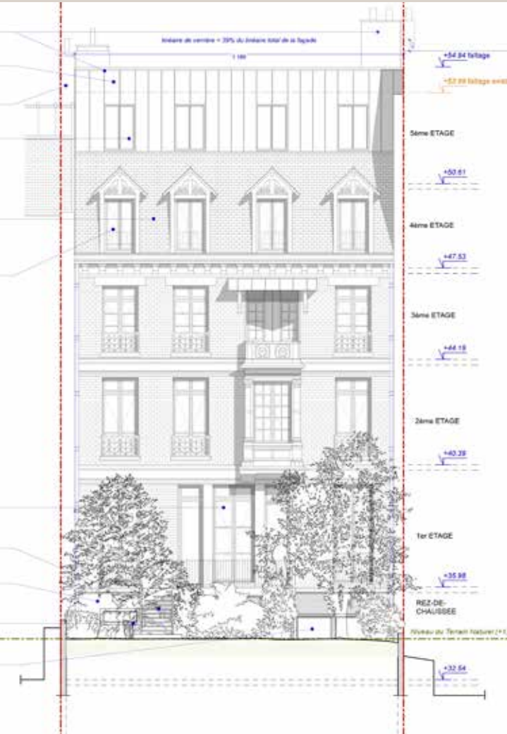
Élévation de la façade côté jardin du corps de logis principal, nouveau projet (© Fabrice Drain architecte).
