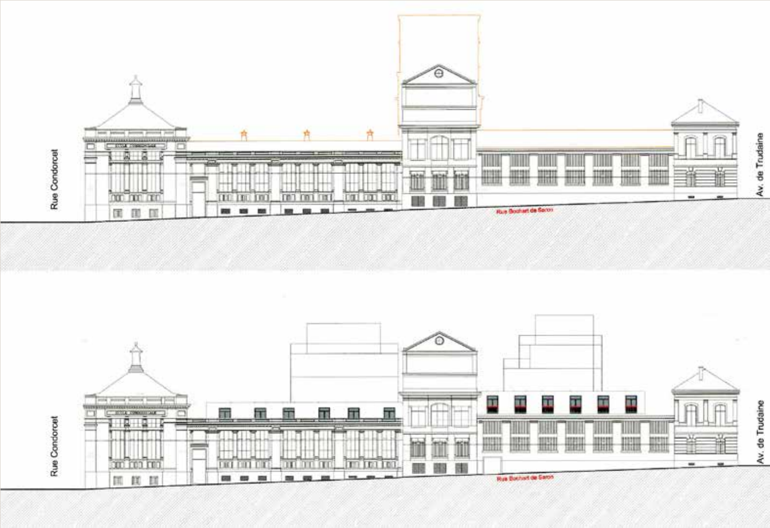
Élévation de la façade sur la rue Bochard-de-Saron, états existant (en haut) et projeté (en bas) (© DVA).
