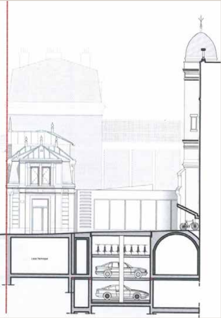
Coupe longitudinale, projet présenté en mai 2017 (© Fabrice Drain architecte).
