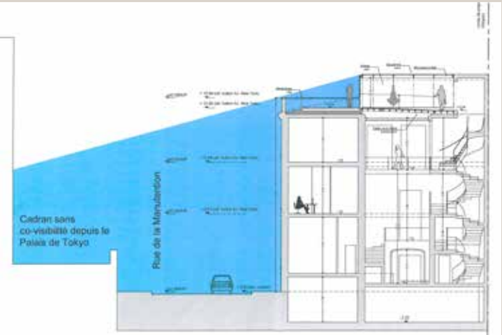
Coupe longitudinale projetée présentant la surélévation et le prolongement de l’escalier (© Patrick Le Priol).
