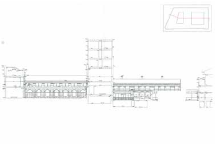
Coupe longitudinale, état existant (© DVA).
