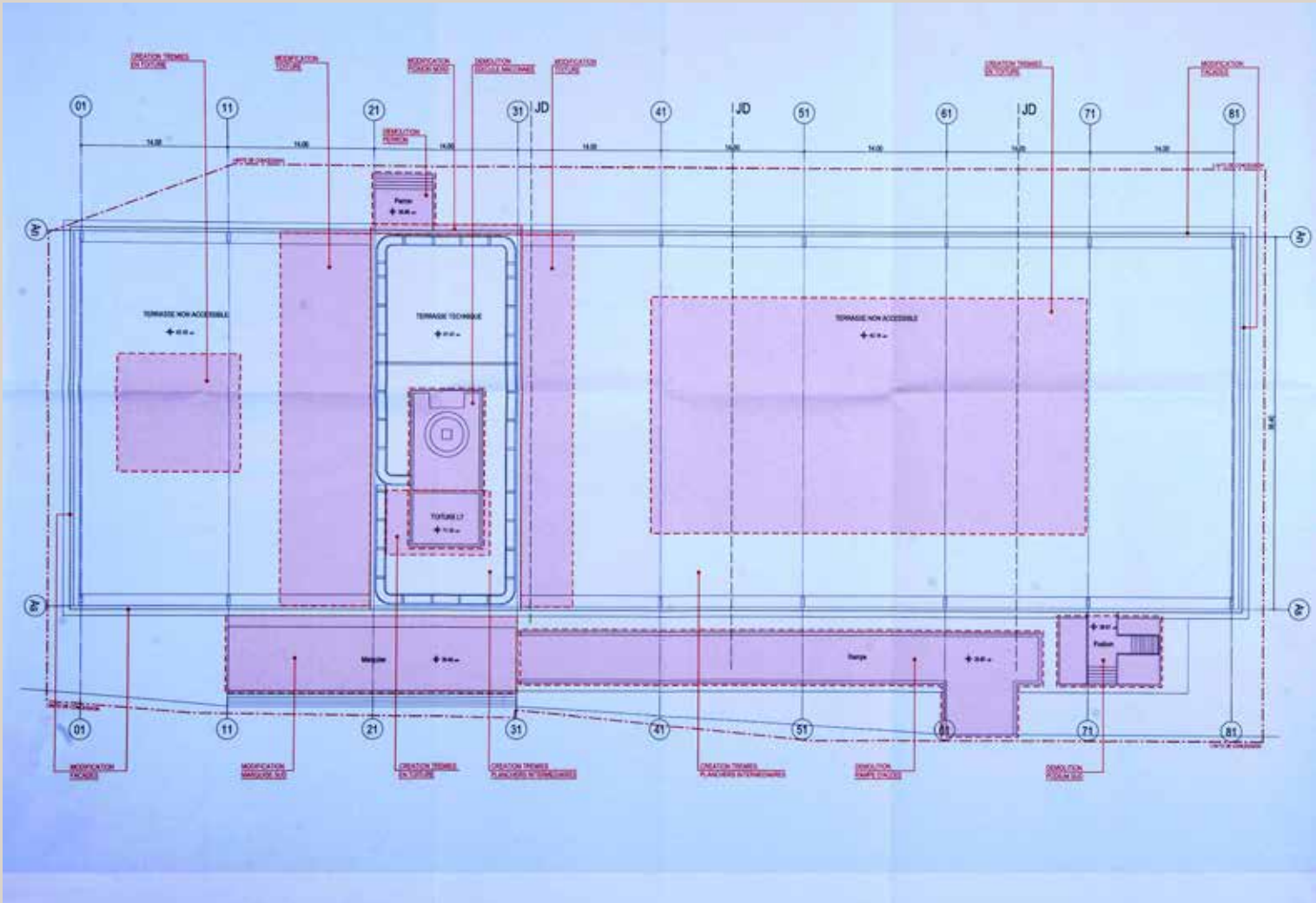
Plan masse des constructions dont la démolition est projetée (© Gehry & partners et Agence Search).
