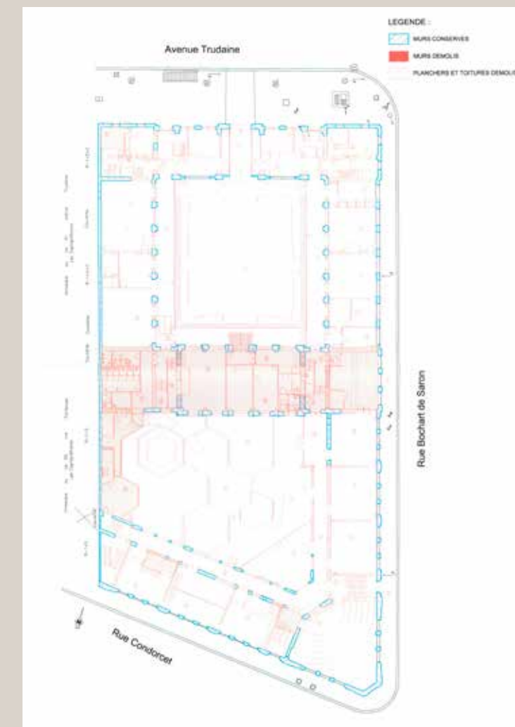
Plan actuel du rez-de-chaussée, présentant en rouge les démolitions envisagées (© DVA).
