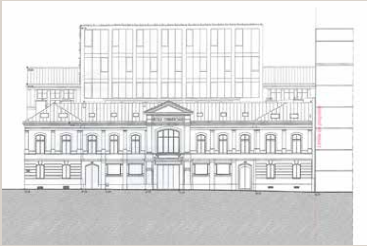
Élévation de la façade sur l'avenue Trudaine, état projeté (© DVA).
