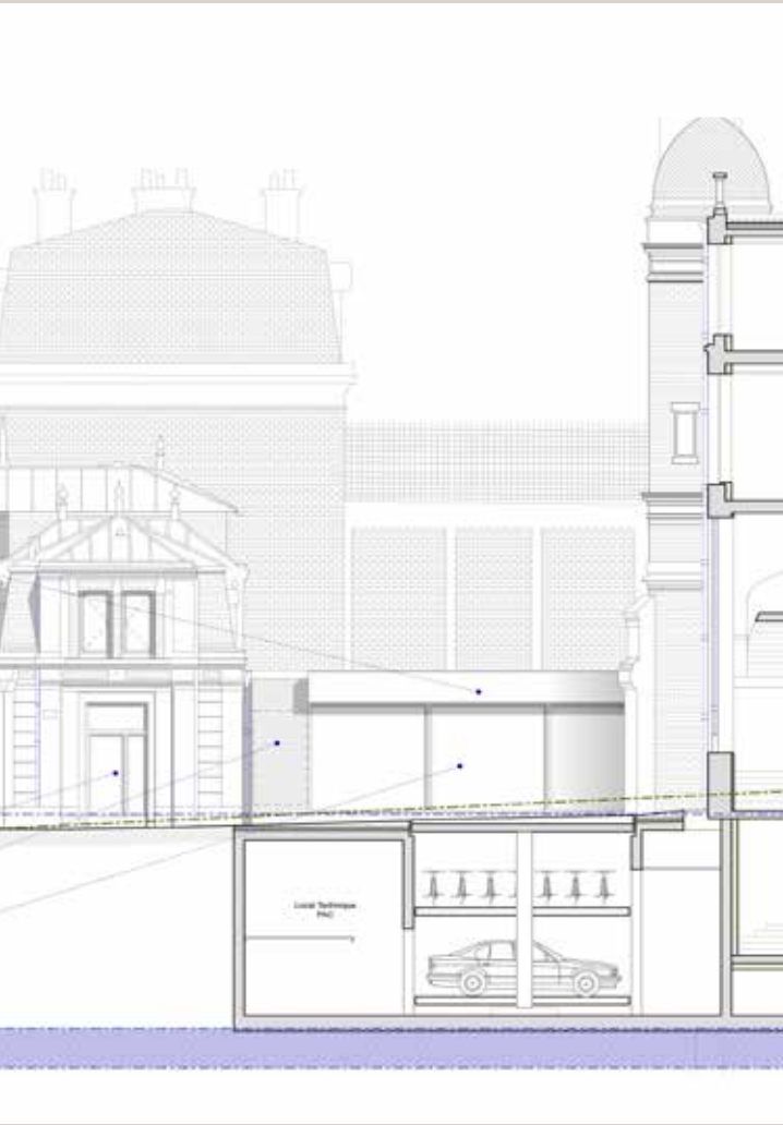
Coupe longitudinale, nouveau projet (© Fabrice Drain architecte).
