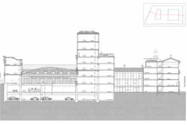
Coupe longitudinale, état projeté (© DVA).
