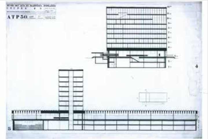
Coupes transversale et longitudinale, 14 janvier 1957 (© IFA).
