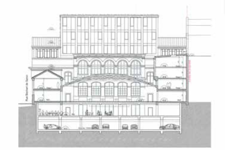
Coupe transversale de l’immeuble central, état projeté (© DVA).
