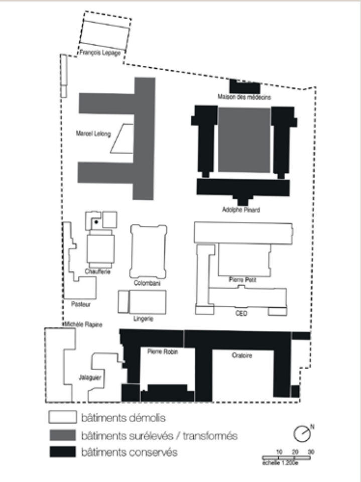
Plan du site présentant les modifications et démolitions projetées (© Anyoji Beltrando).
