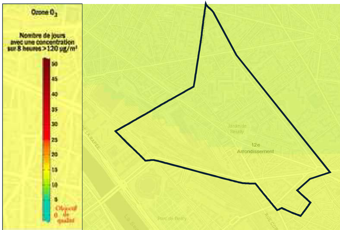
Carte annuelle de pollution à l'ozone – année 2019 Nombre de jours supérieurs à 120µg/m³ pour 8 heures
