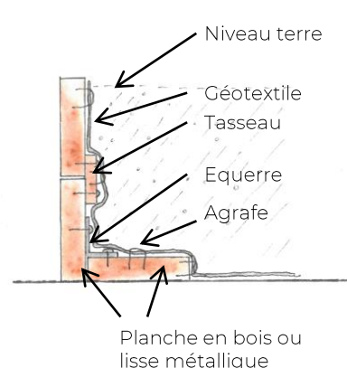
Coupe de principe de fixation pour planche
