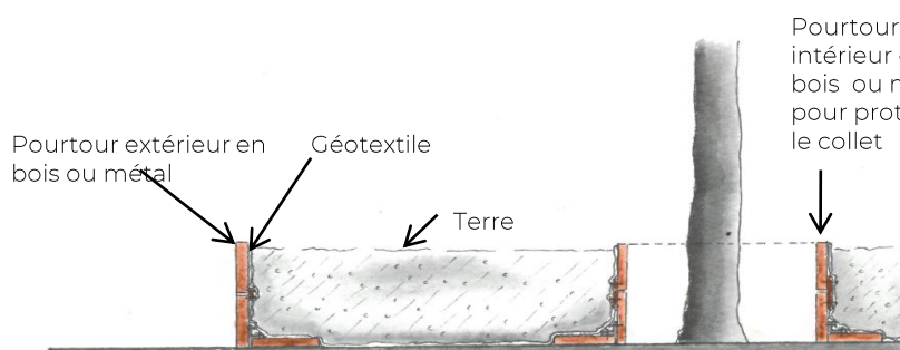
Coupe de principe d'un entourage
