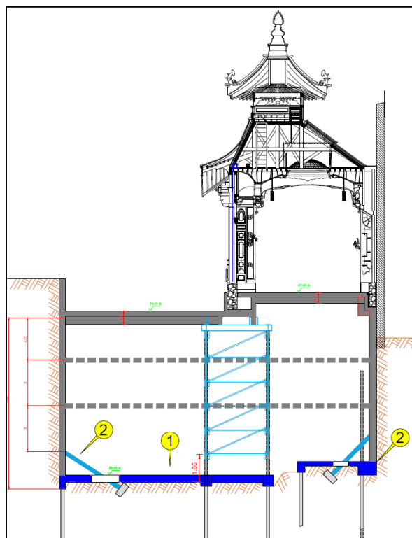
Réalisation du radier
