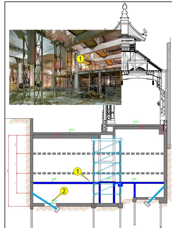
Réalisation des nouveaux niveaux de plancher
