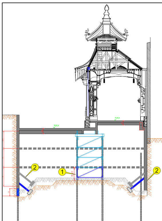
Fin du terrassement Rabattement de nappe
