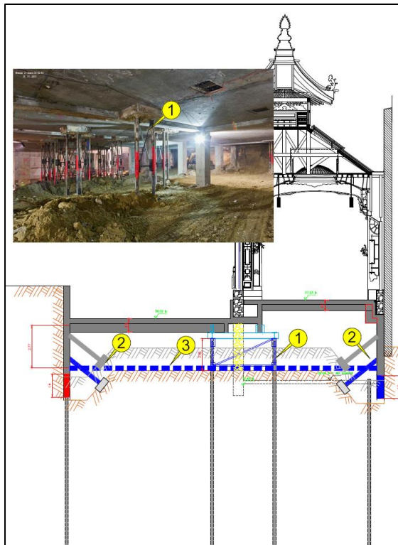
Terrassement et voile par passe en taupe
