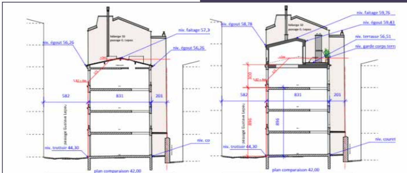
Coupe, état existant (à gauche) et projeté (à droite) (© VN architecte).
