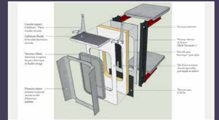
Schéma présentant le principe de la rénovation thermique des façades (© Patriarche architectes).
