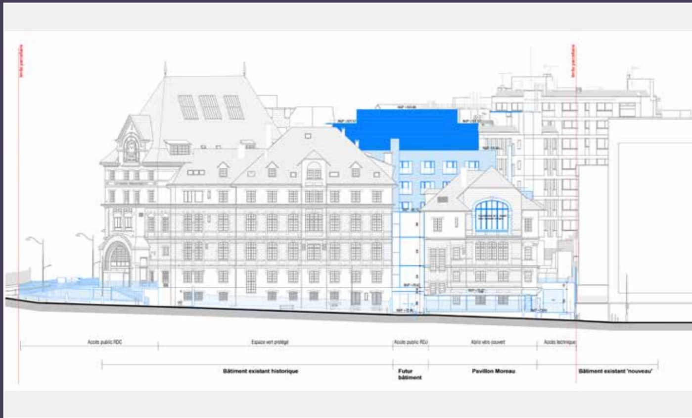
Élévation des façades sur l'avenue Mathurin-Moreau, état projeté (en bleu les nouvelles réalisations) (© Brunet-Saunier Architecture).
