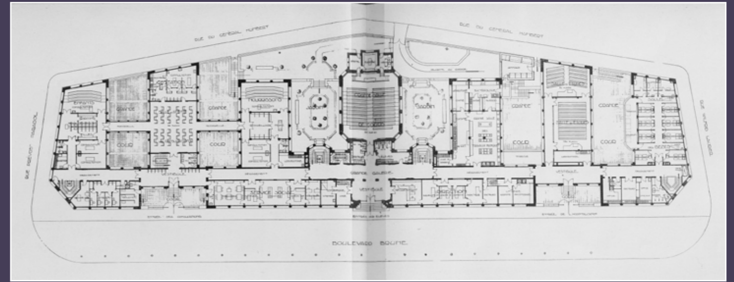
Plan du rez-de-chaussée, publiée dans L'Architecture , n° 10, 1933.
