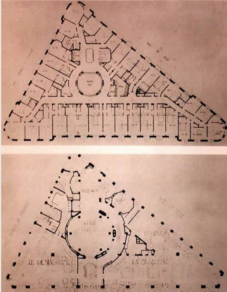
Plans de l'hôtel de Paris. De bas en haut: rez-de-chaussée, 2 e étage. Hôtels de voyageurs , Paris, Ed. Ch. Moreau, s.d. [1930], 2 e vol. pl. 14 et 15.
