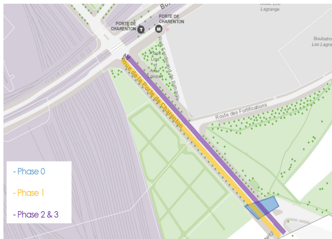
[Phasage détaillé des zones concernées par les travaux]
