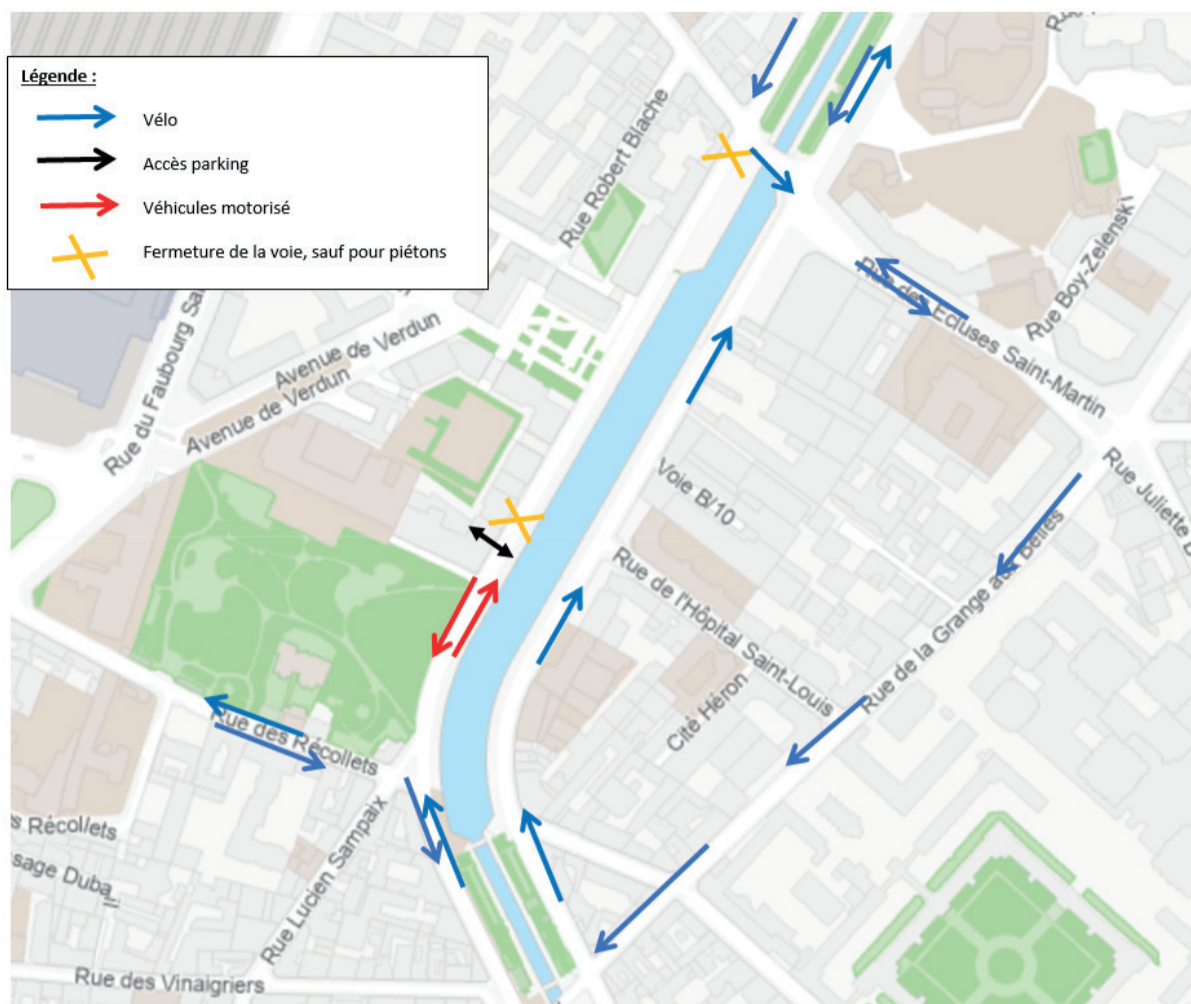
Plan de déviation du chantier
