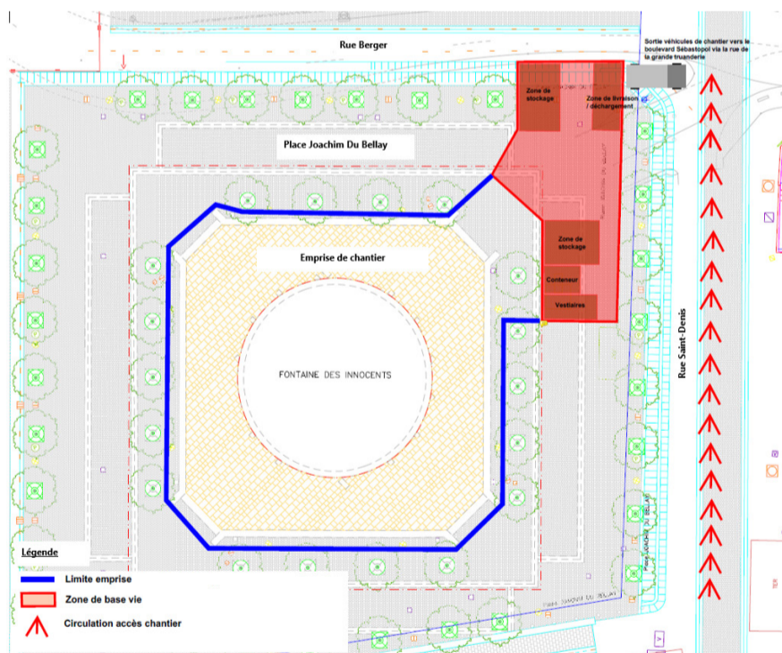
Schéma de l'emprise du chantier
