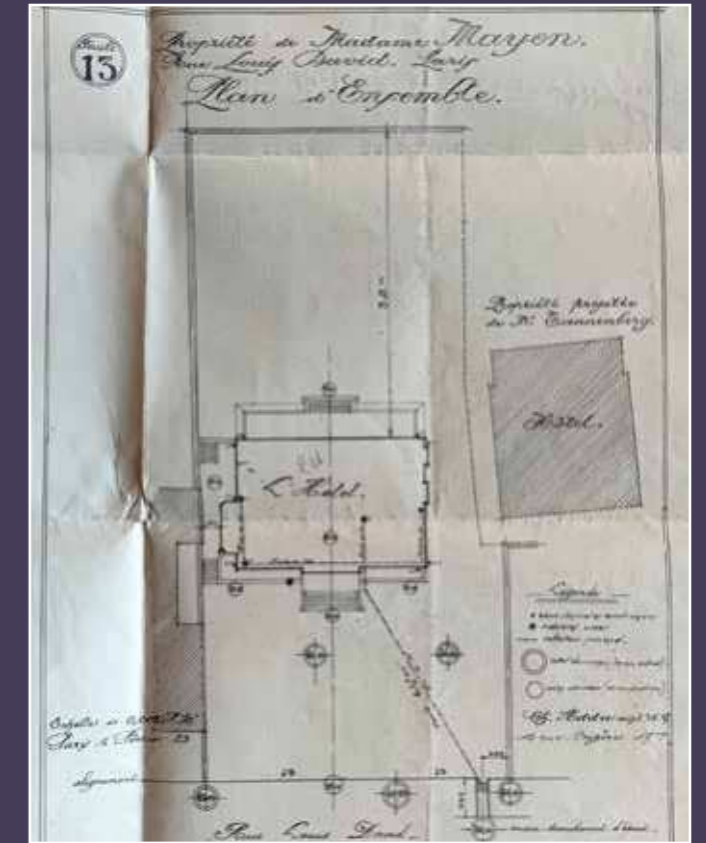
Charles Adda, architecte, plan de l'hôtel particulier au 13-15 rue Louis David pour Mme Mayen, 1923 (AD75).
