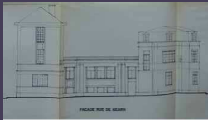
Jacques Vial, architecte, élévation sur la rue de Béarn, état avant projet, 1989 (AD75).
