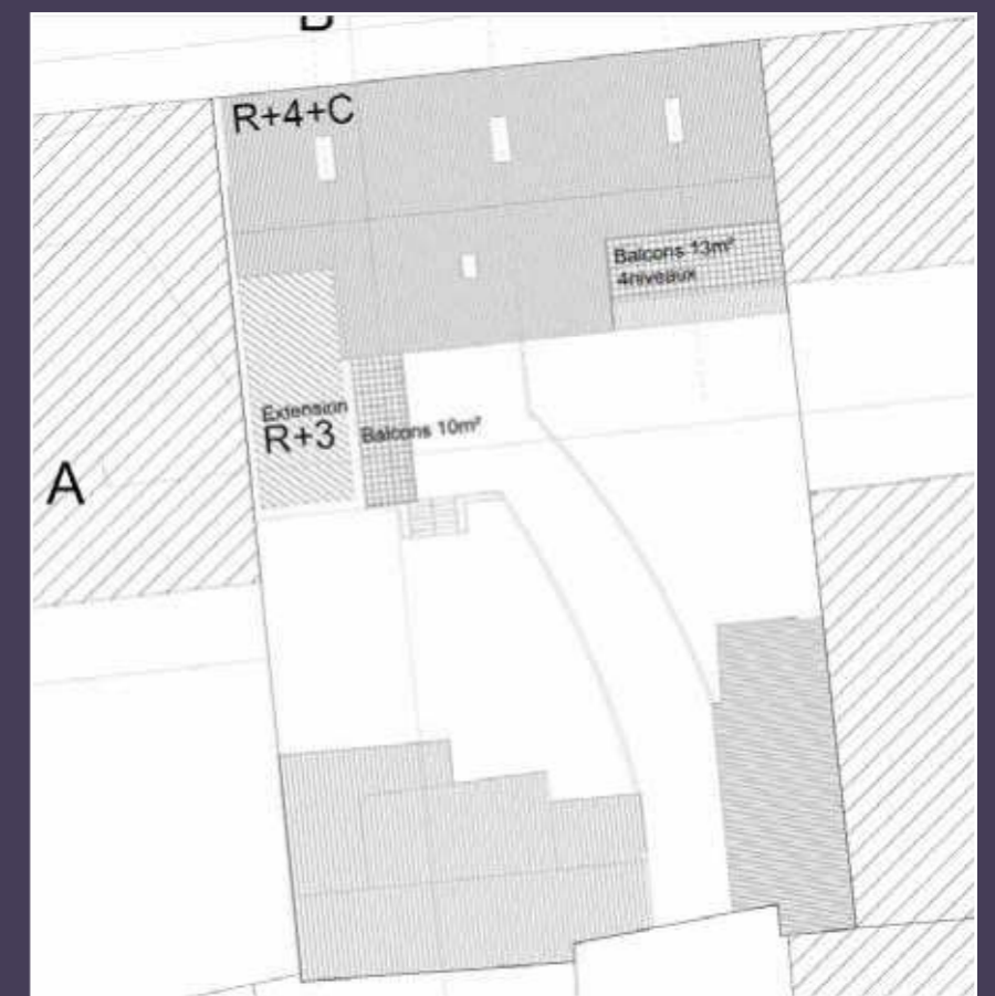
Premier projet d'épaississement du bâtiment sur rue (© 3F).
