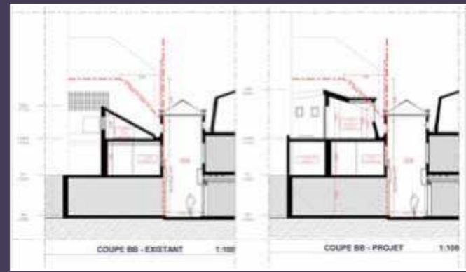
Coupe BB, état existant et projet (© AHA!).
