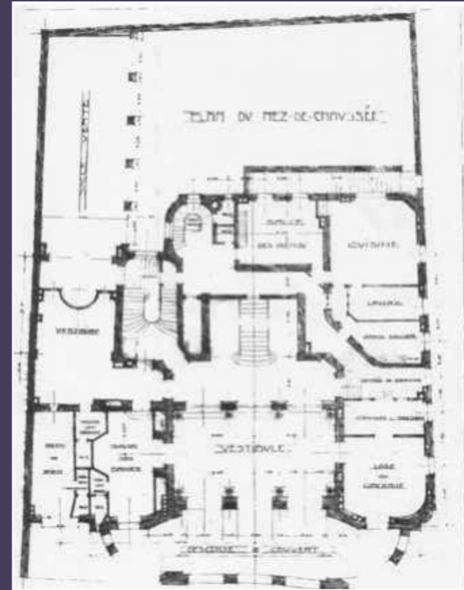
Henri-Paul Nénot, architecte, plan du rez-de-chaussée, 1909 (AD75).
