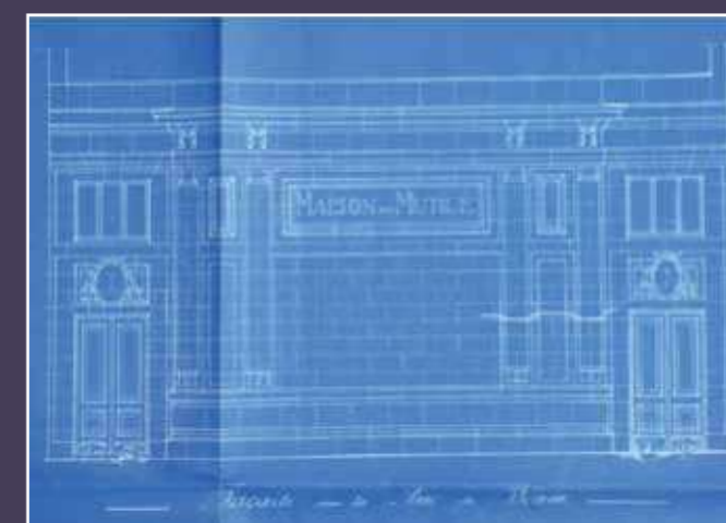
Paul Pelletier, architecte, projet de façade sur la rue de Béarn, 1920 (AD75).
