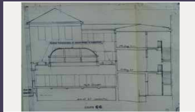
Jacques Vial, architecte, coupe sur l'ancienne cour, état avant projet, 1989 (AD75).
