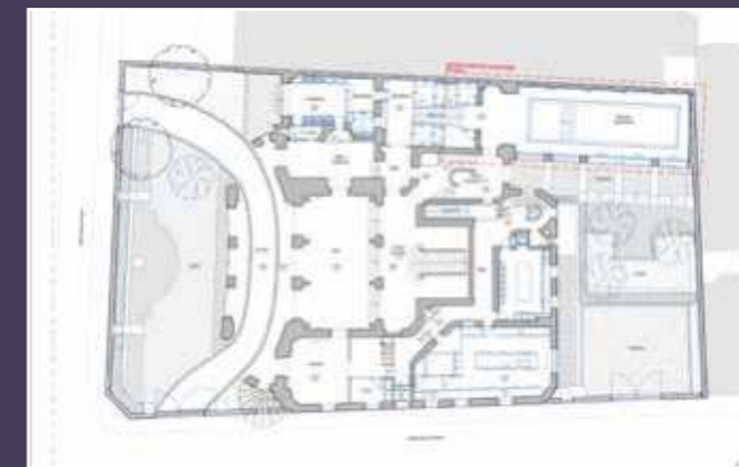
Plan du rez-de-chaussée, état projeté (© LBBA Architecture).
