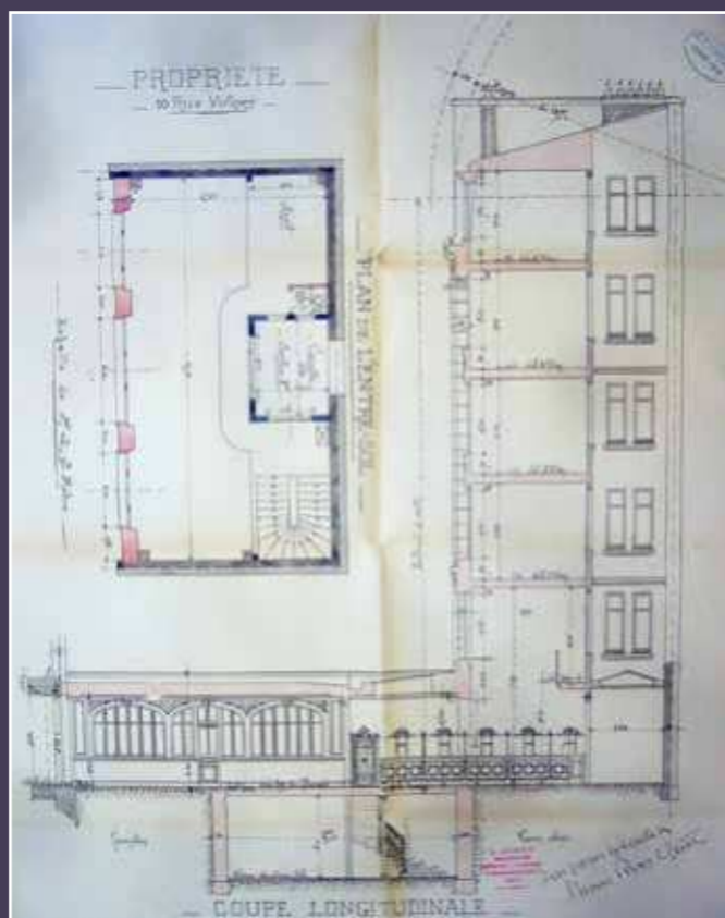
Louis Girod, architecte, plan de l'entresol et coupe longitudinale, mars 1919 (AD75).
