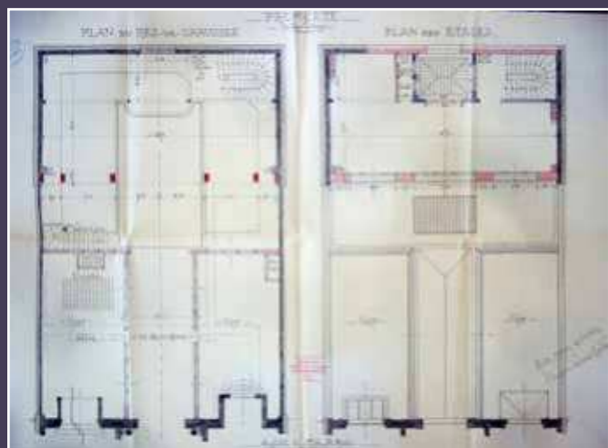
Louis Girod, architecte, plan du rez-de-chaussée et des étages du bâtiment situé en fond de parcelle, mars 1919 (AD75).
