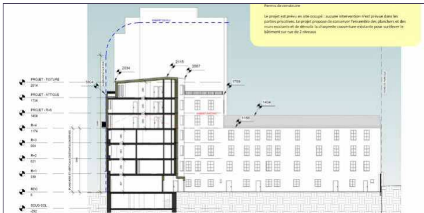
Coupe longitudinale, nouveau projet (© Atelier LA architectes).
