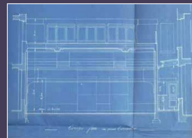
Paul Pelletier, architecte, coupe sur la nouvelle aile et salle projetées, 1920 (AD75).
