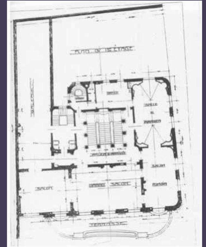
Henri-Paul Nénot, architecte, plan du premier étage, 1909 (AD75).
