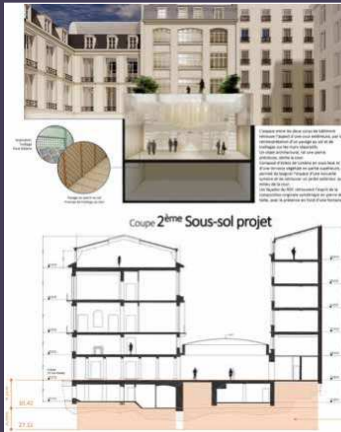
Coupe transversale d'insertion du projet et coupe projetée du deuxième sous-sol (© Moatti - Rivière).
