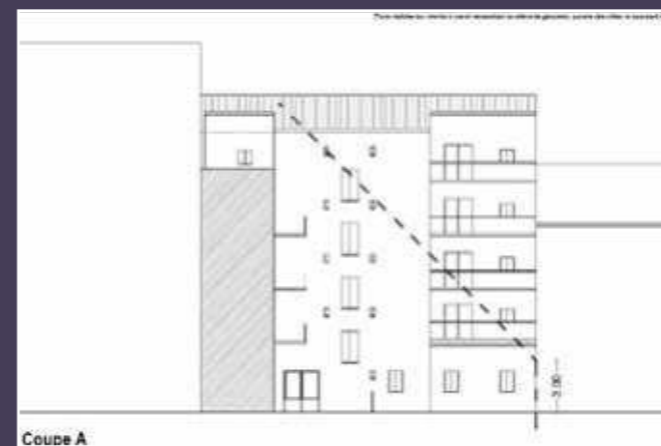
Coupe du bâtiment sur rue projeté, première version (© 3F).
