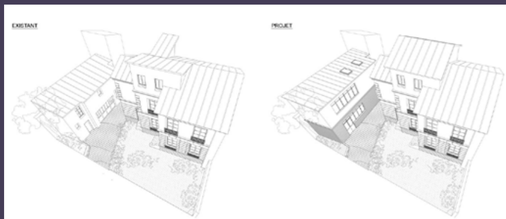
Axonométrie montrant le pavillon et le bâtiment des communs, état existant (à gauche) et projet (à droite) (© 3F/MAP architecture).
