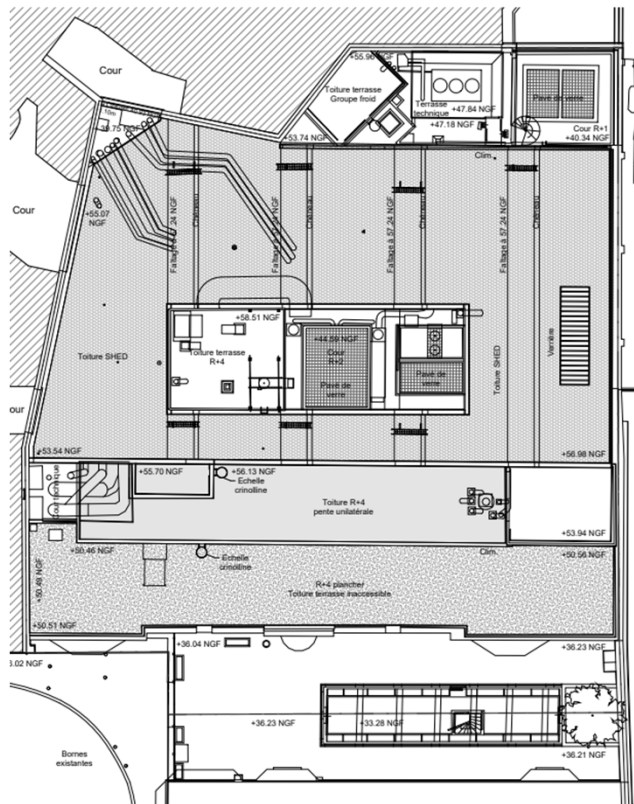
EXISTANT
