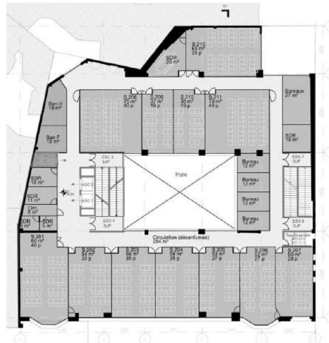
PLAN PROJET
