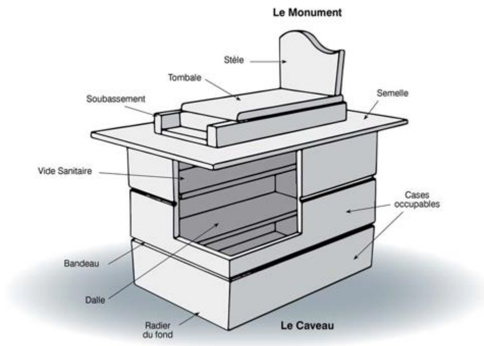
Schéma d'un monument et de son caveau
