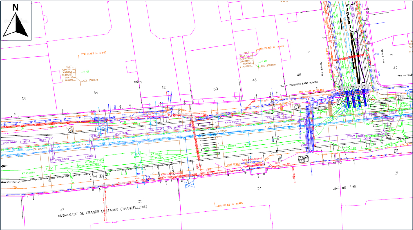
Extrait du plan de synthèse des réseaux
