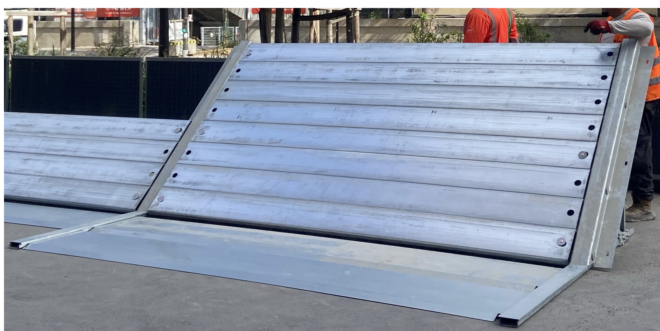
Une barrière anti-crues - Crédits : Ville de Paris
